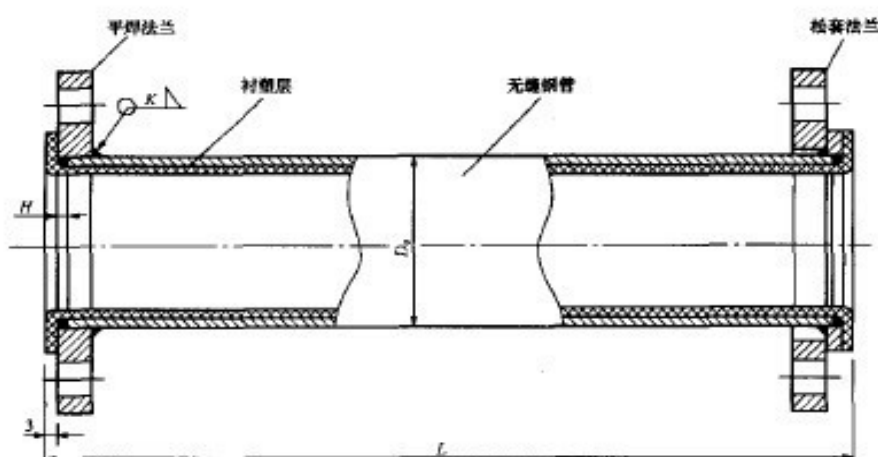
图 A.1 钢塑复合管
