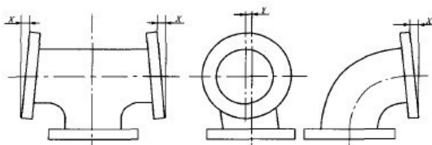
图 C.1 管件的形位公差
