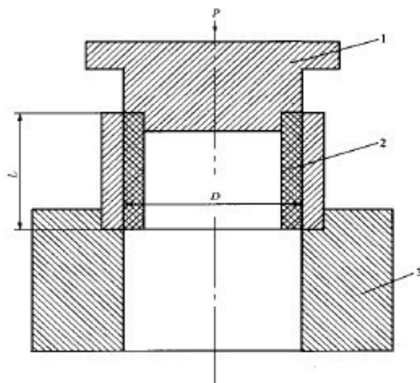
1—压头；2—复合管；3—托模
