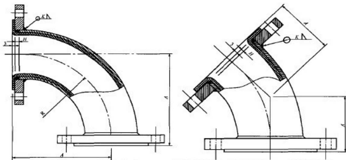
图 A.2 钢塑复合管件（90° 弯头、45° 弯头）
